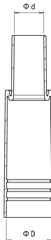
断面 A-A
